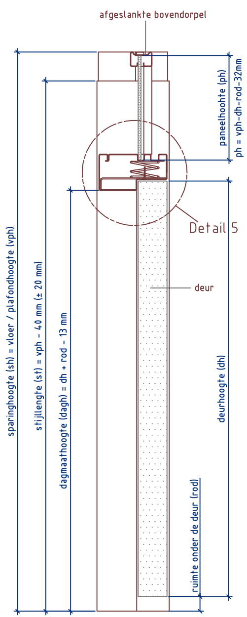
Doorsnede BB
